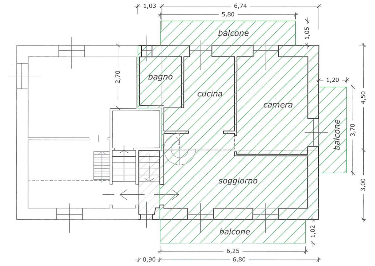
PIANO PRIMO
